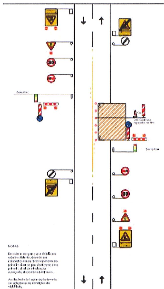
Figura n.º 3 – Trabalhos na Rua D. Vasco da Gama, com circulação alternada sinalização luminosa
