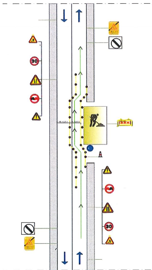
Figura n.º 1 – Fase 1 dos trabalhos na Avenida da República com estreitamento da via
